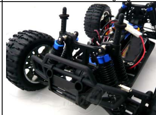
8 Öldruckstoßdämpfer
