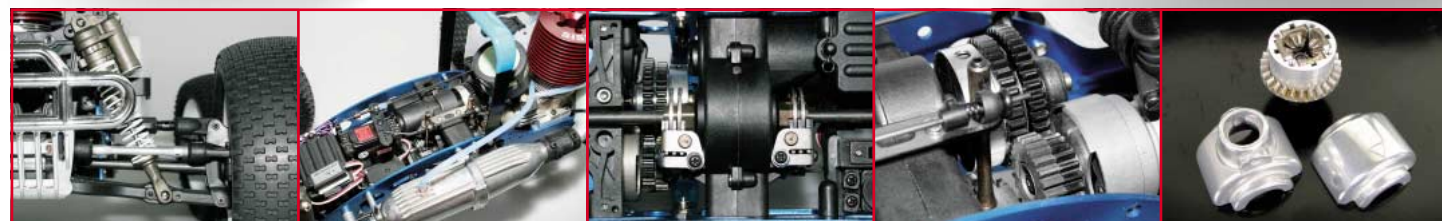
verstärkter Antriebsstrang
